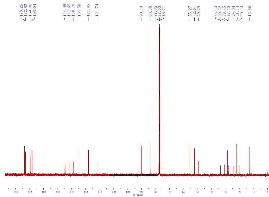
附 3b : ^{13}\text{C} -NMR (100 MHz, \text{CDCl}_3 )
