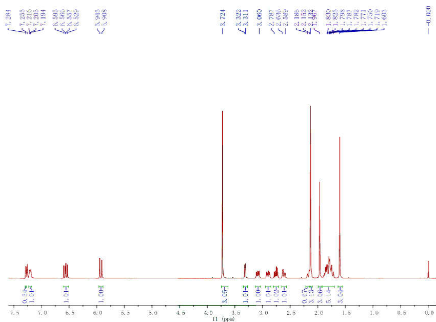
附 3a : ^1\text{H} -NMR (400 MHz, \text{CDCl}_3 )
