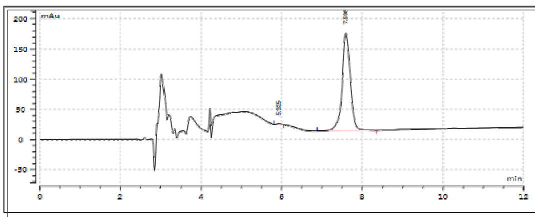
峰列表
