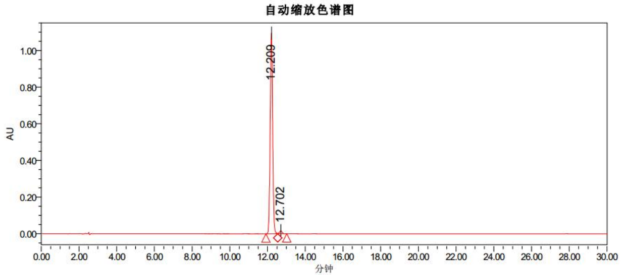
峰结果
